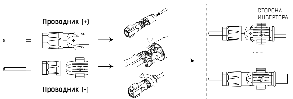
Рисунок 3.4.7 Инструкция по монтажу кабелей
