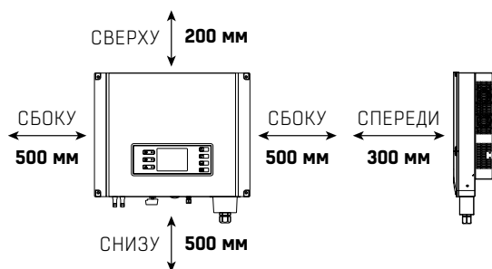
Рисунок 3.4.3. Расстояния до места установки инвертора
