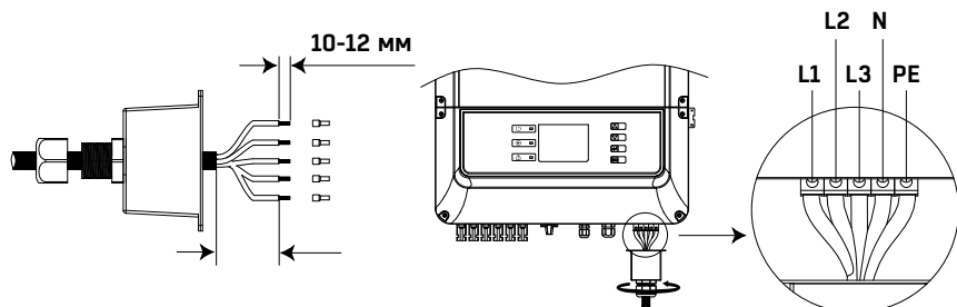
Рисунок 3.4.6 Подключение инвертора к сети
