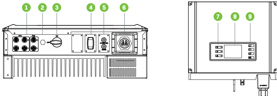
Рисунок 2.3.1 Схема инвертора
