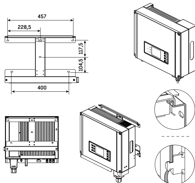
Рисунок 3.4.4 Инструкция по креплению инвертора на поверхность
