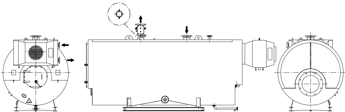
Рис. 17 Конденсационный экономайзер
