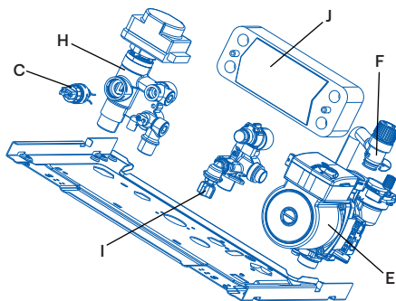
Двухконтурные котлы: GreenLine S 2.20/2.26/2.30/2.35TW
