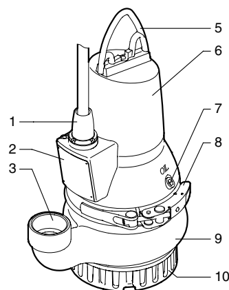
Рис. 1 Насос DP 10.50
