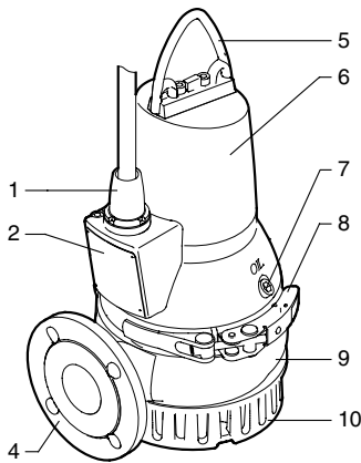
Рис. 2 Насос DP 10.65
