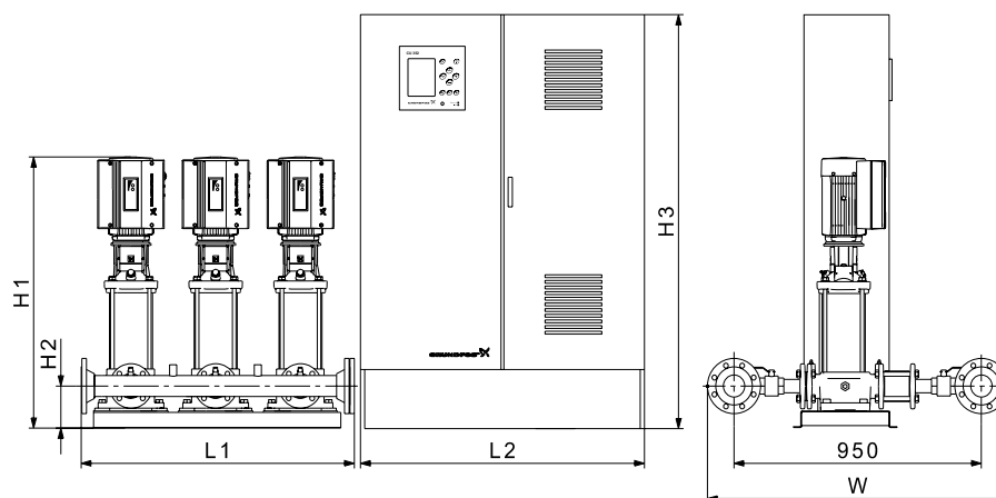
Рис. 61 Размерная схема установки повышения давления Hydro MPC со шкафом управления, смонтированным на полу (исполнение С). Установка повышения давления приведена в качестве примера. Входящие в поставку насосы могут отличаться от показанных на схеме.
