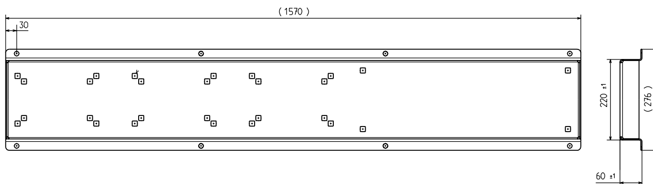
Рис. 96 Рама-основание
