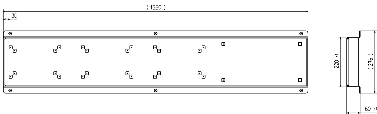
Рис. 93 Рама-основание
