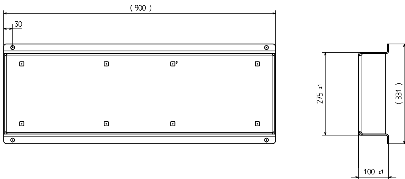
Рис. 92 Рама-основание
