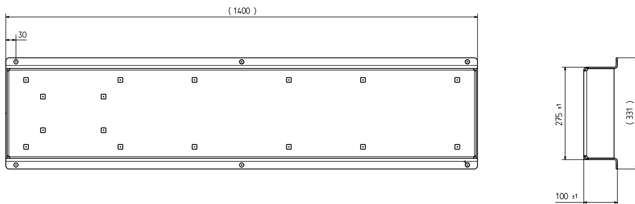
Рис. 98 Рама-основание
