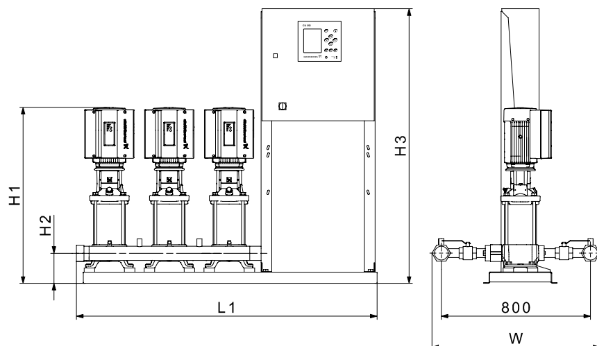
Рис. 57 Размерная схема установки повышения давления Hydro MPC со шкафом управления, который смонтирован на одной раме-основании с насосами (исполнение A). Установка повышения давления приведена в качестве примера. Входящие в поставку насосы могут отличаться от показанных на схеме.
