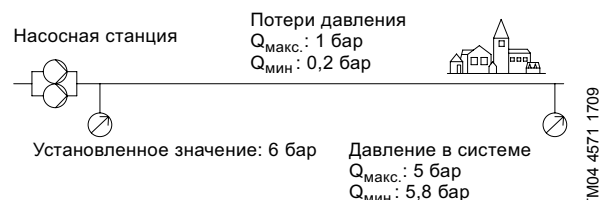
Рис. 29 Без пропорционального регулирования давления
