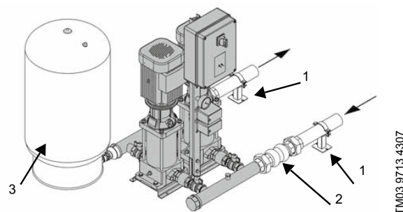
Рис. 130 Пример установки с резиновыми вибровставками и опорами для труб (стандартный объем поставки Grundfos обозначен серым цветом)
