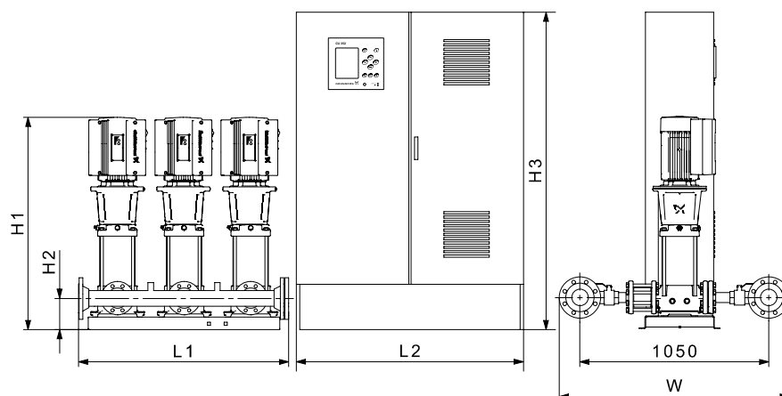
Рис. 65 Размерная схема установки повышения давления Hydro MPC со шкафом управления, смонтированным на полу (исполнение C). Установка повышения давления приведена в качестве примера. Входящие в поставку насосы могут отличаться от показанных на схеме.
