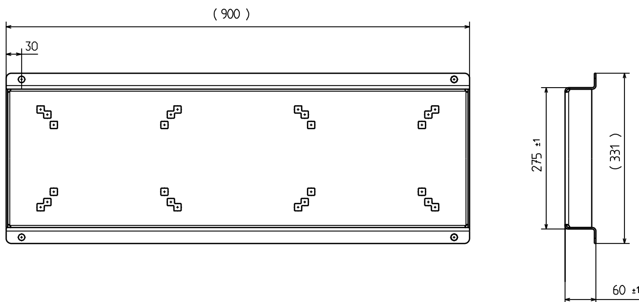
Рис. 89 Рама-основание
