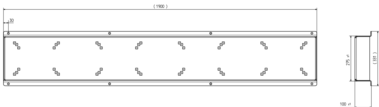
Рис. 101 Рама-основание
