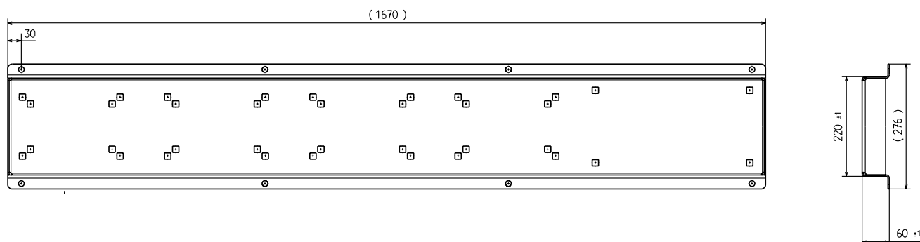
Рис. 99 Рама-основание
