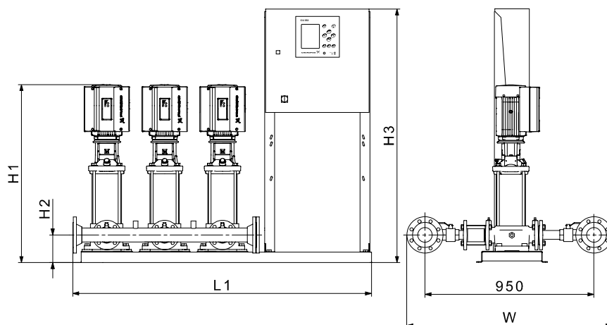
Рис. 60 Размерная схема установки повышения давления Hydro MPC со шкафом управления, который смонтирован на одной раме-основании с насосами (исполнение А). Установка повышения давления приведена в качестве примера. Входящие в поставку насосы могут отличаться от показанных на схеме.
