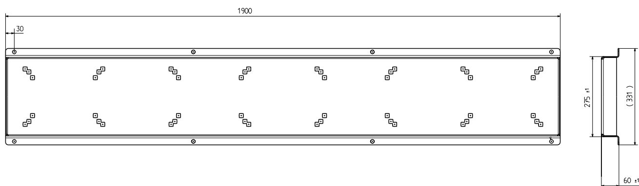
Рис. 100 Рама-основание
