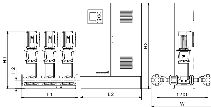
Рис. 50 Размерная схема установки повышения давления Hydro MPC со шкафом управления, смонтированным на полу (исполнение C). Установка повышения давления приведена в качестве примера. Входящие в поставку насосы могут отличаться от показанных на схеме.
