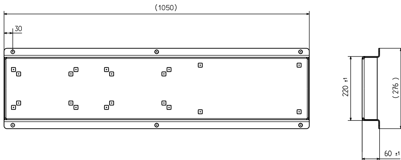
Рис. 88 Рама-основание
