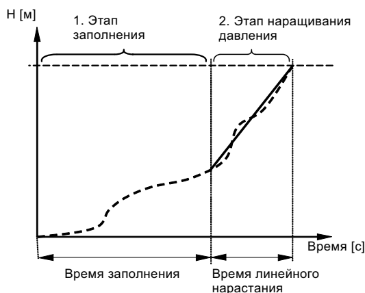
Рис. 113 Этапы заполнения и нарастания давления
