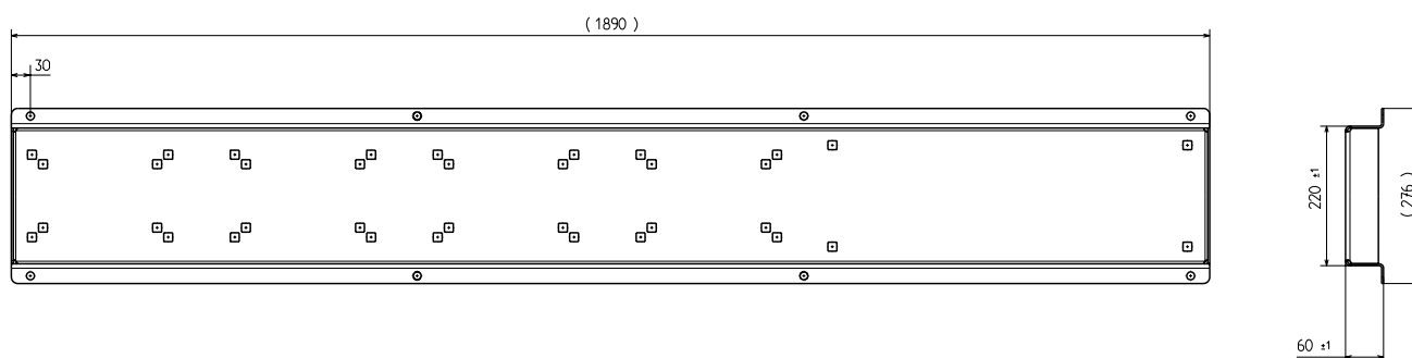
Рис. 103 Рама-основание
