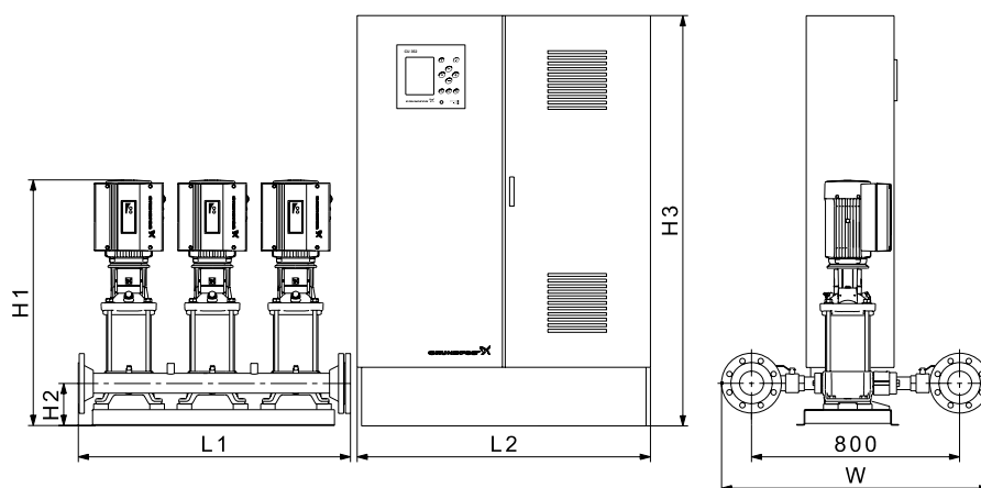
Рис. 58 Размерная схема установки повышения давления Hydro MPC со шкафом управления, смонтированным на полу (исполнение C). Установка повышения давления приведена в качестве примера. Входящие в поставку насосы могут отличаться от показанных на схеме.
