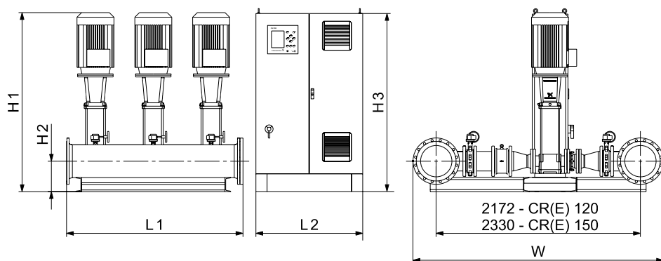
Рис. 52 Размерная схема установки повышения давления Hydro MPC со шкафом управления, смонтированным на отдельной раме-основании (исполнение D). Установка повышения давления приведена в качестве примера. Входящие в поставку насосы могут отличаться от показанных на схеме.
