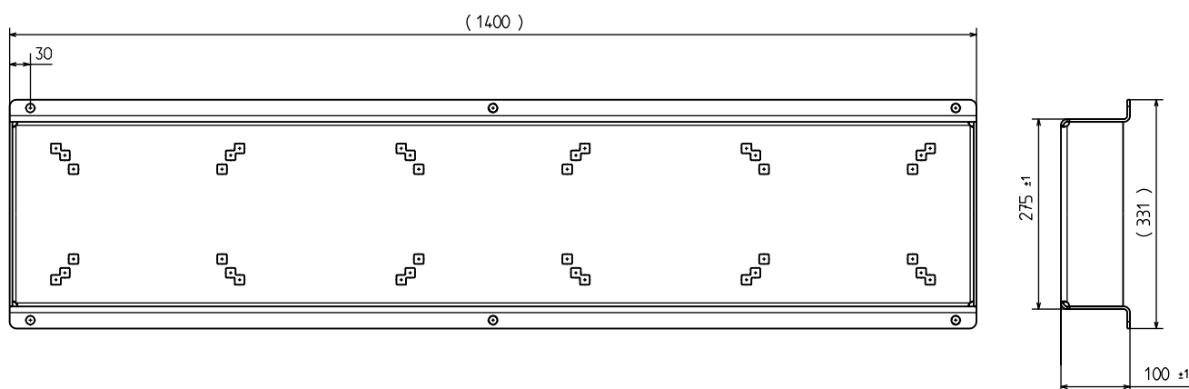
Рис. 95 Рама-основание
