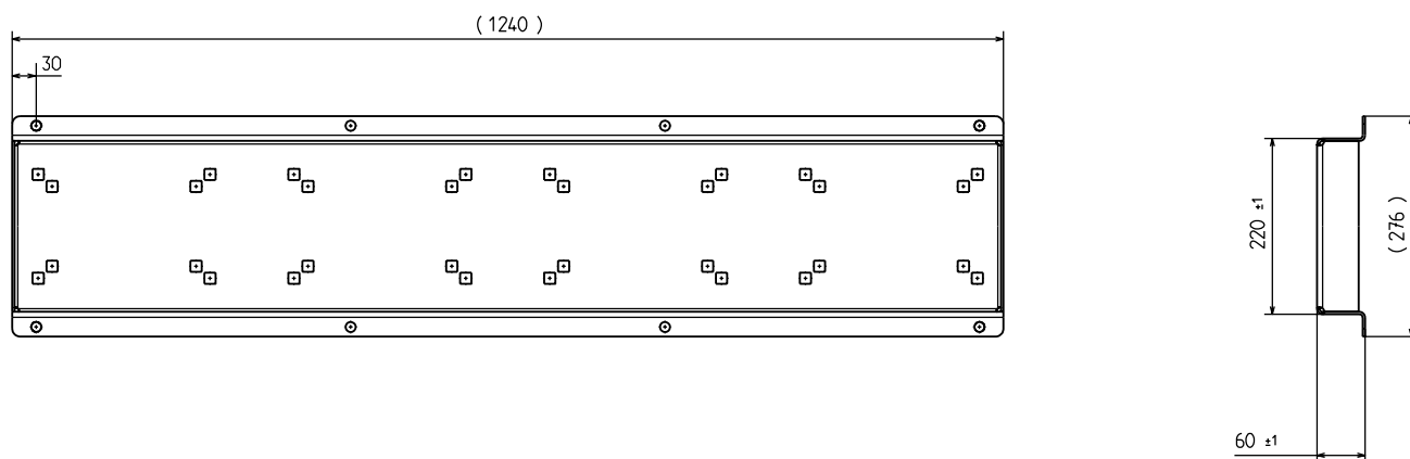
Рис. 102 Рама-основание
