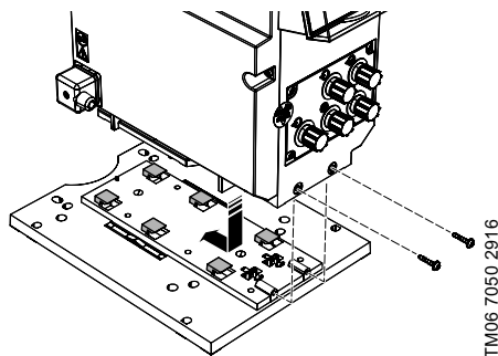
5-сур. Сорғыны монтаждық тақтаға орнату
