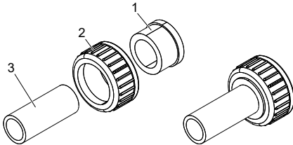
8-сур. Жабыстыру (дәнекерлеу) бойынша гидравликалық қосылулар
