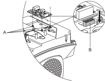
Рис. 66 Установка модуля СИМ
