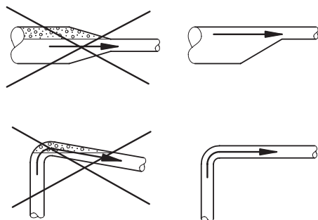
Рис. 4 Установка всасывающего трубопровода Минимальный диаметр скважины 100 мм (4"), см. рис. 5.
