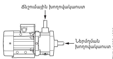
Նկար 6 Ներմղման և ճնշամղման խողովակաոստեր
