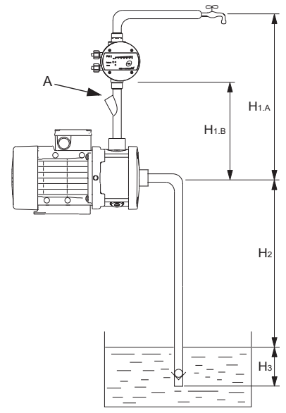
Նկար 7 Ինքաններմող պոմպի համար խորհուրդ տրվող խողովակաշարերը
