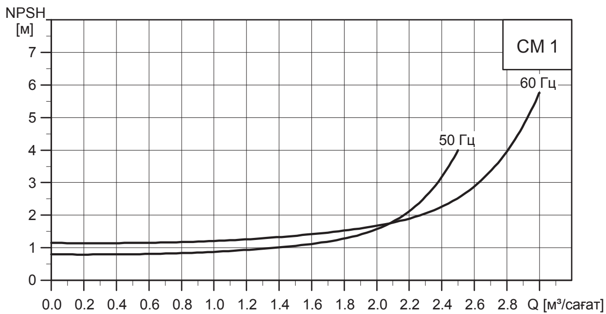
21-сур. CM 1 үшін қисық NPSH
