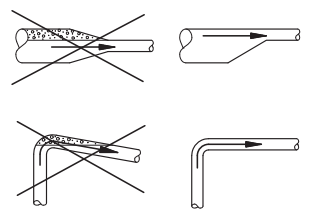
Նկար 5 Խողովակաշար
