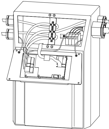
Рис. 3 Подключение электропитания
