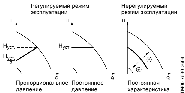
Рис. 8 Регулируемый и нерегулируемый режимы
