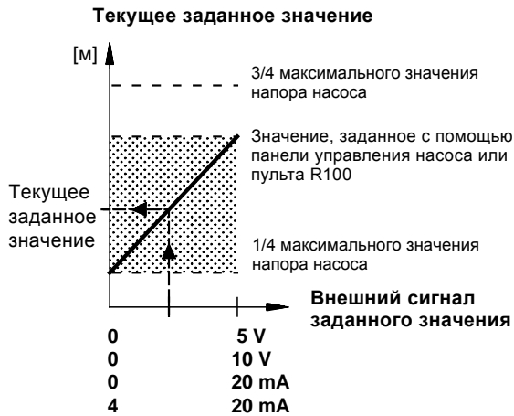
Рис. 17 Зависимость между фактическим значением и внешним сигналом заданного значения при режиме эксплуатации с пропорциональным регулированием давления
