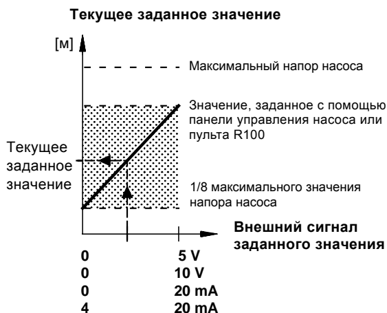
Рис. 18 Зависимость между фактическим значением и внешним сигналом заданного значения при регулировании постоянного давления
