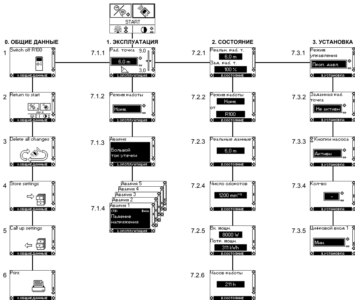
Рис. 15 Пульт R100 обменивается информацией с насосом через инфракрасный порт
