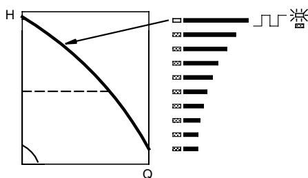
Рис. 13 Макс. характеристика
