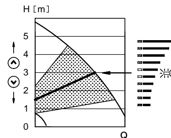
Рис. 11 Насос с пропорционально регулируемым давлением
