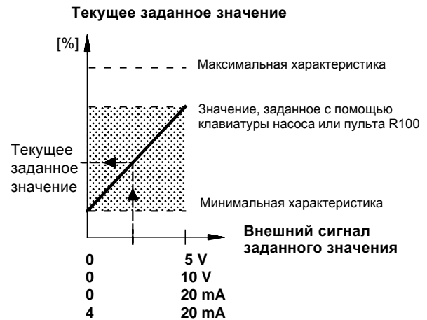
Рис. 19 Зависимость между фактическим значением и внешним сигналом заданного значения при режиме эксплуатации с постоянной характеристикой
