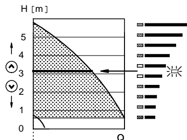
Рис. 12 Насос с регулированием постоянного давления
