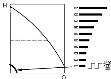
Рис. 14 Мин. характеристика
