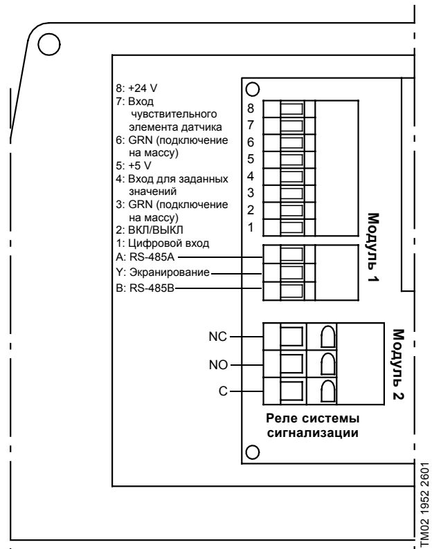
Рис. 4 Схема соединений
