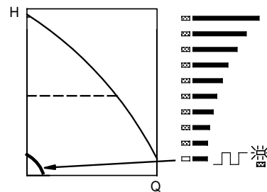
Рис. 19 Мин. характеристика
