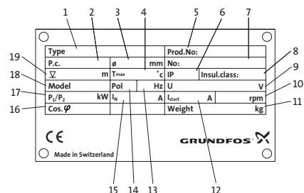
Рис. 2 Фирменная табличка с номинальными параметрами
