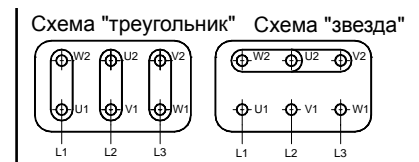
Рис. 8 Клеммы для подключения электропитания
