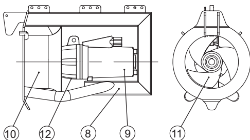
Рис. 1 Насос модели SRP
