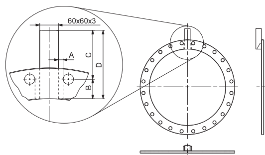
Рис. 5 Основа крепления на соединительном фланце
