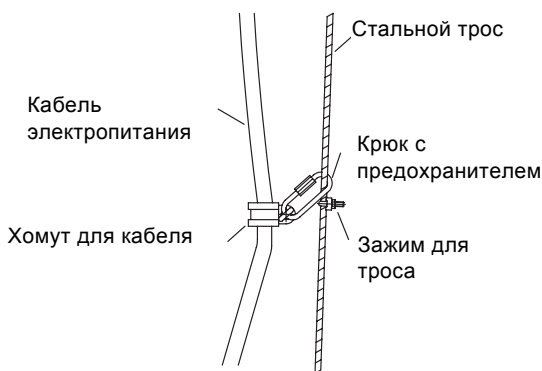
Рис. 7 Кабель электропитания и стальной трос
