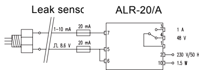
Рис. 10 Датчик протечек и реле ALR-20/A
