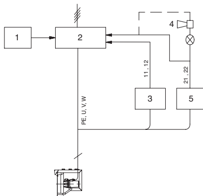
Рис. 13 Блок-схема
