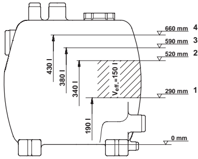
Рис. 5 Разные уровни жидкости в сборном резервуаре
