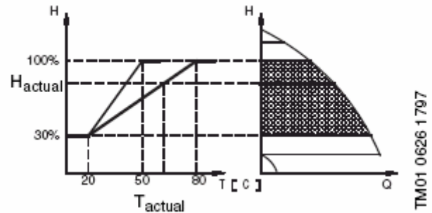
Рис. 7 Регулирование по температуре
