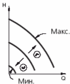
Рис. 5 Рабочие характеристики
