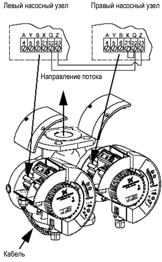
Рис. 8 Сдвоенные насосы с модулем GENI
