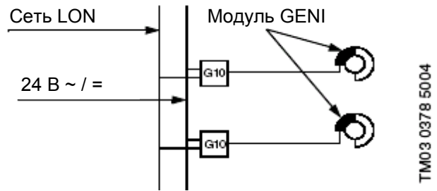
Рис. 10 Подключение к сети модуля LON
