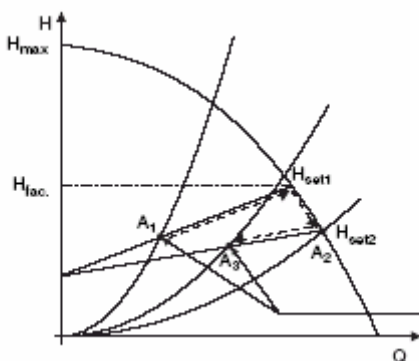
Рис. 3 Функция "AUTO ADAPT "
