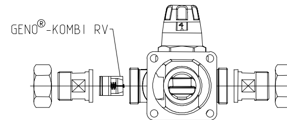
Рис. 1.2: Монтаж обратного клапана GENO®-KOMBI-RV (принадлежности)
