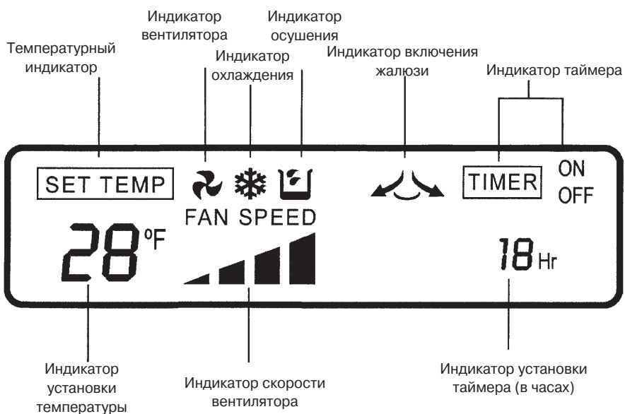
Рис.5.2 - Жидкокристаллический дисплей
