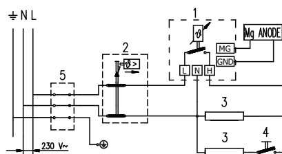
Электросхема
