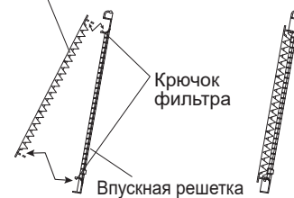
Воздушный фильтр
