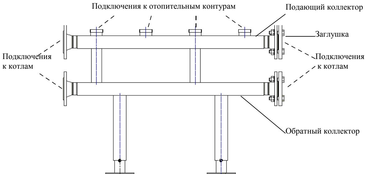
Рис. 2. 2-х контурный коллектор Ду50
