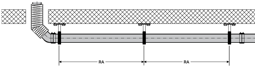
Рисунок 37: Расстояние между точками крепления по горизонтали
