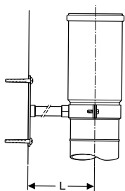
Рисунок 6: Неподвижная опора
