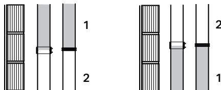
Рисунок 59: Переход с электромуфтой Geberit или стыковой сваркой
