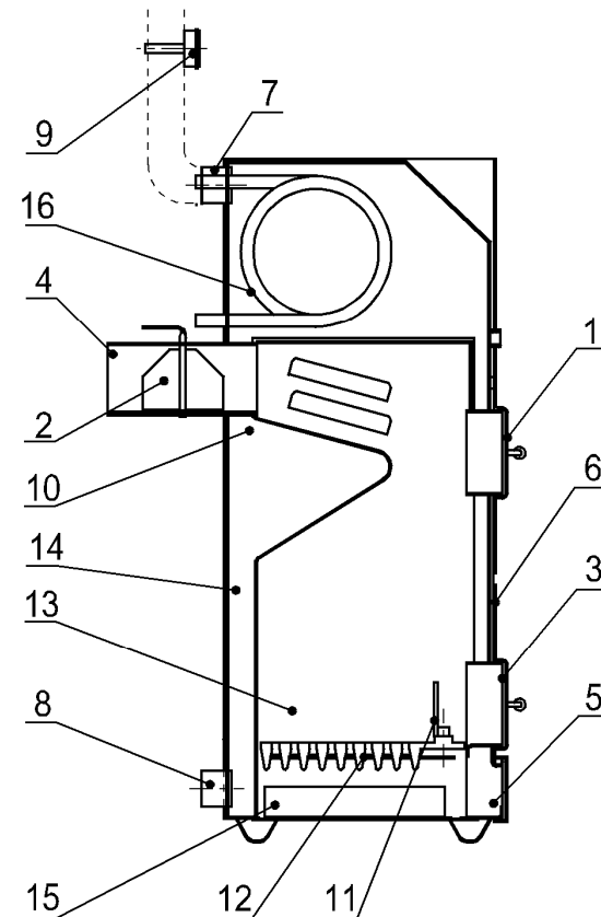
Рис.3 Устройство котла КСТГВ
