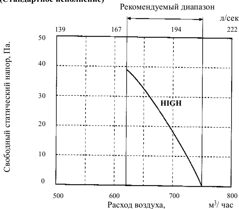
Рис. 48 Зависимость расхода воздуха и свободного статического напора вентилятора
