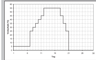
Aufheizprogramm 6
