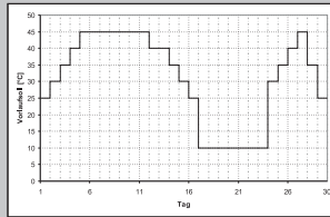
Aufheizprogramm 4:
