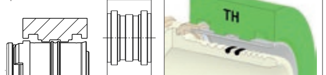
Контур обжима TH: прочие изготовители
