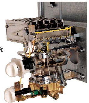
Газово-гидравлический блок
