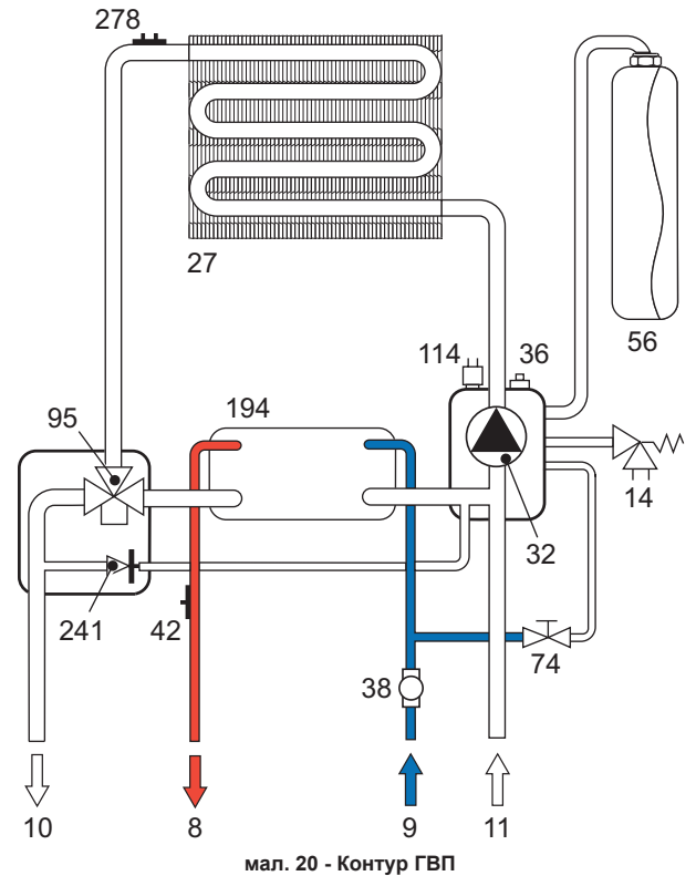
мал. 20 - Контур ГВП
