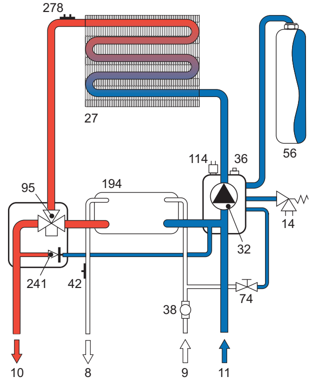
мал. 19 - Контур опалення
