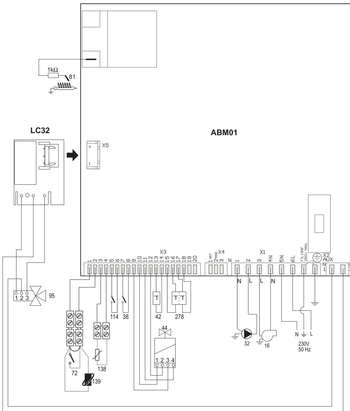
рис. 21 - Электрическая система
