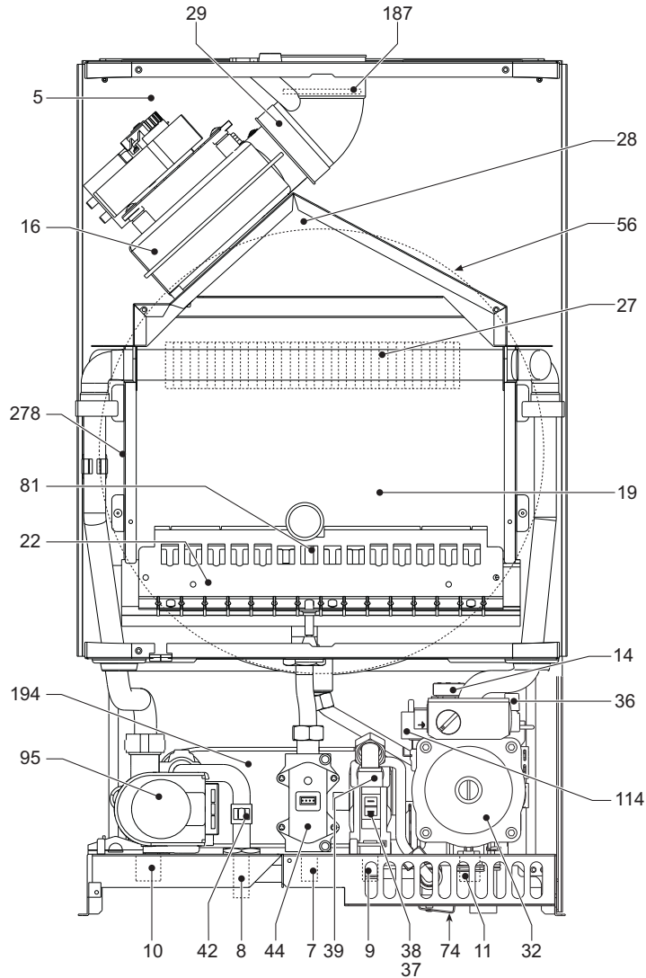
мал. 18 - Загальний вигляд
