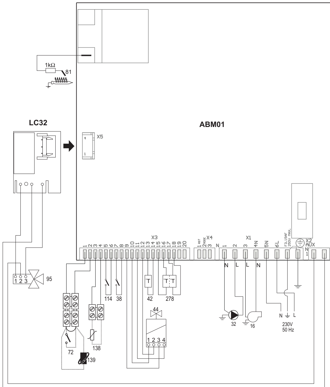
мал. 21 - Електрична схема
