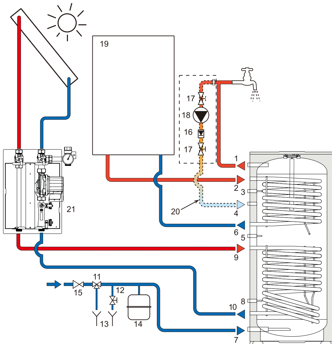
Рис. 4 – Гидравлический контур ECOUNTIT N 2C
