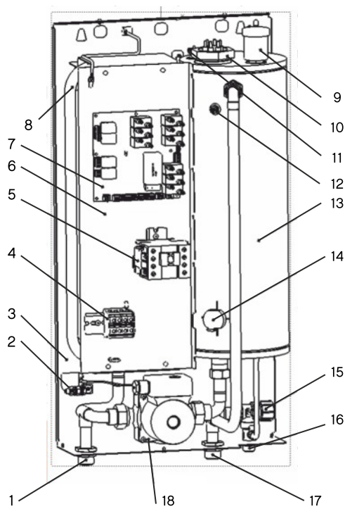
Устройство прибора
