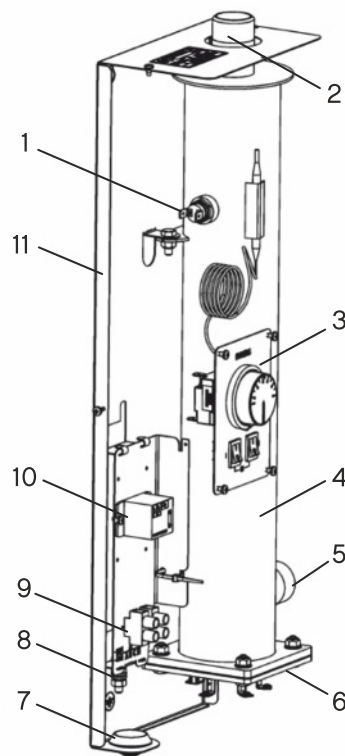
Устройство прибора
