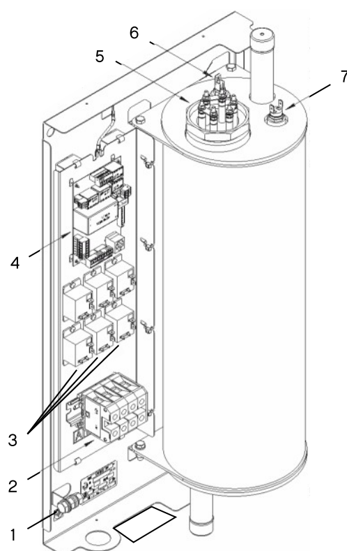
Устройство прибора
