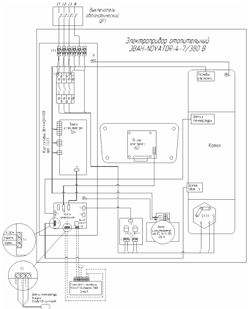
Рисунок 7 Схема подключения ЭВАН NOVATOR -4-7/ 380 В
