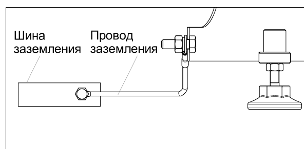
Рисунок 3. Электромонтаж провода заземления
