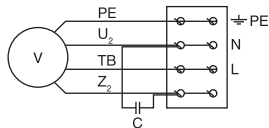
Схема №1 (230 В, 1 фаза)
