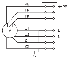
Схема №2 (230 В, 1 фаза)
