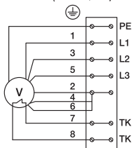
Схема №4 (400 В, 3 фазы)
