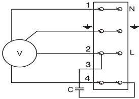
Схема №5 (230 В, 1 фаза)
