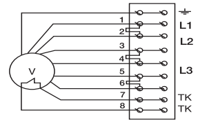
Схема №6 (400 В, 3 фазы)
