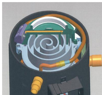
Рис 2: Порты впрыска пара и трубные соединения в спиральном блоке
