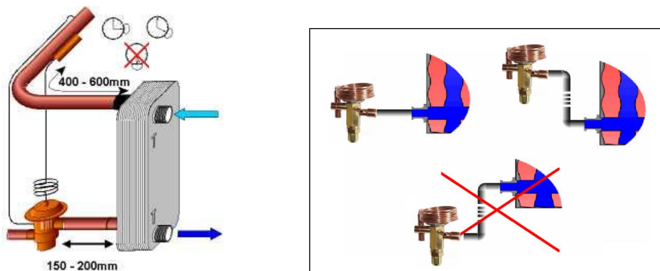
Рис 10: Расположение ТРВ и его термобаллона на пластинчатом теплообменнике (© AL и SWEP)
