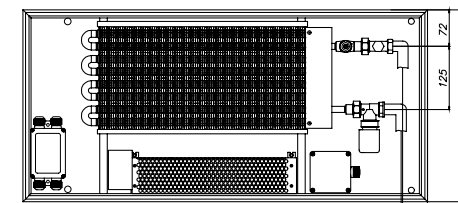
ЕКQ.380.90, вид сбоку
