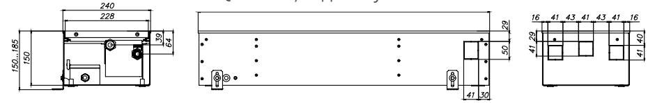
ЕКQ.240.150, вид сбоку
