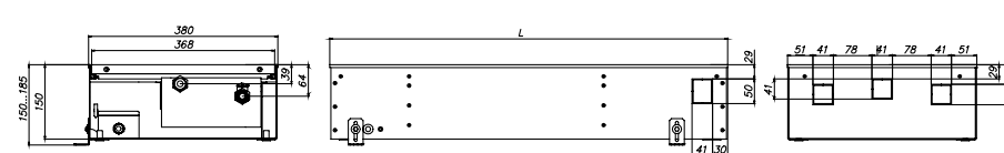
ЕКQ.380.150, вид сбоку
