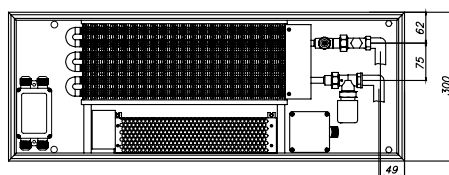
ЕКQ.300.90, вид сбоку
