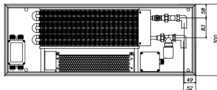
ЕКQ.300.75 вид сбоку
