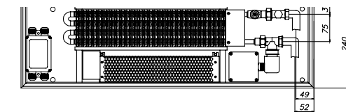
ЕКQ.240.90, вид сбоку
