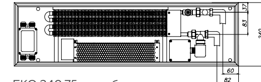
ЕКQ.240.75 вид сбоку
