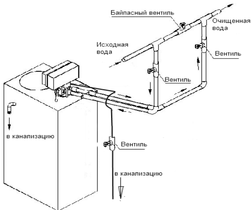
Рисунок 2 – Схема монтажа установки удаления железа и умягчения воды WSDF(C)-1,3-CI-(MIX A) периодического действия типа “Кабинет”
