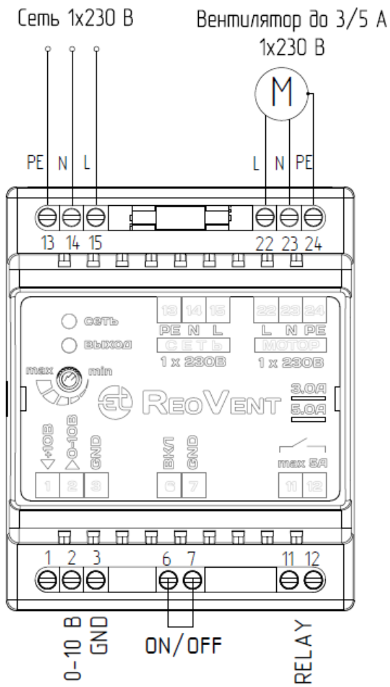
Рис. 3 Подключение регулятора Reovent к шкафу автоматики OPTIBOX
