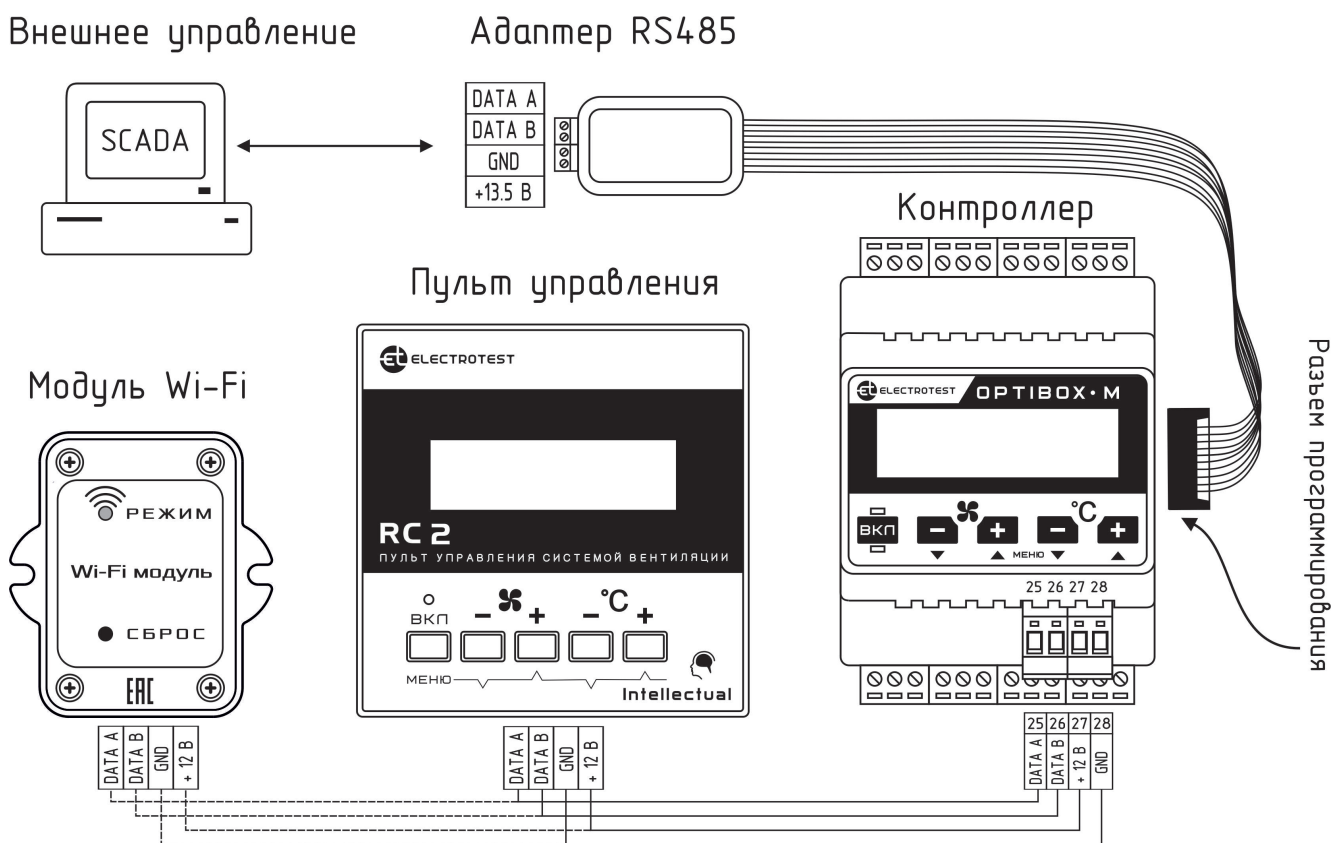
Рис. 2.3 Подключение средств ДУ + SCADA
