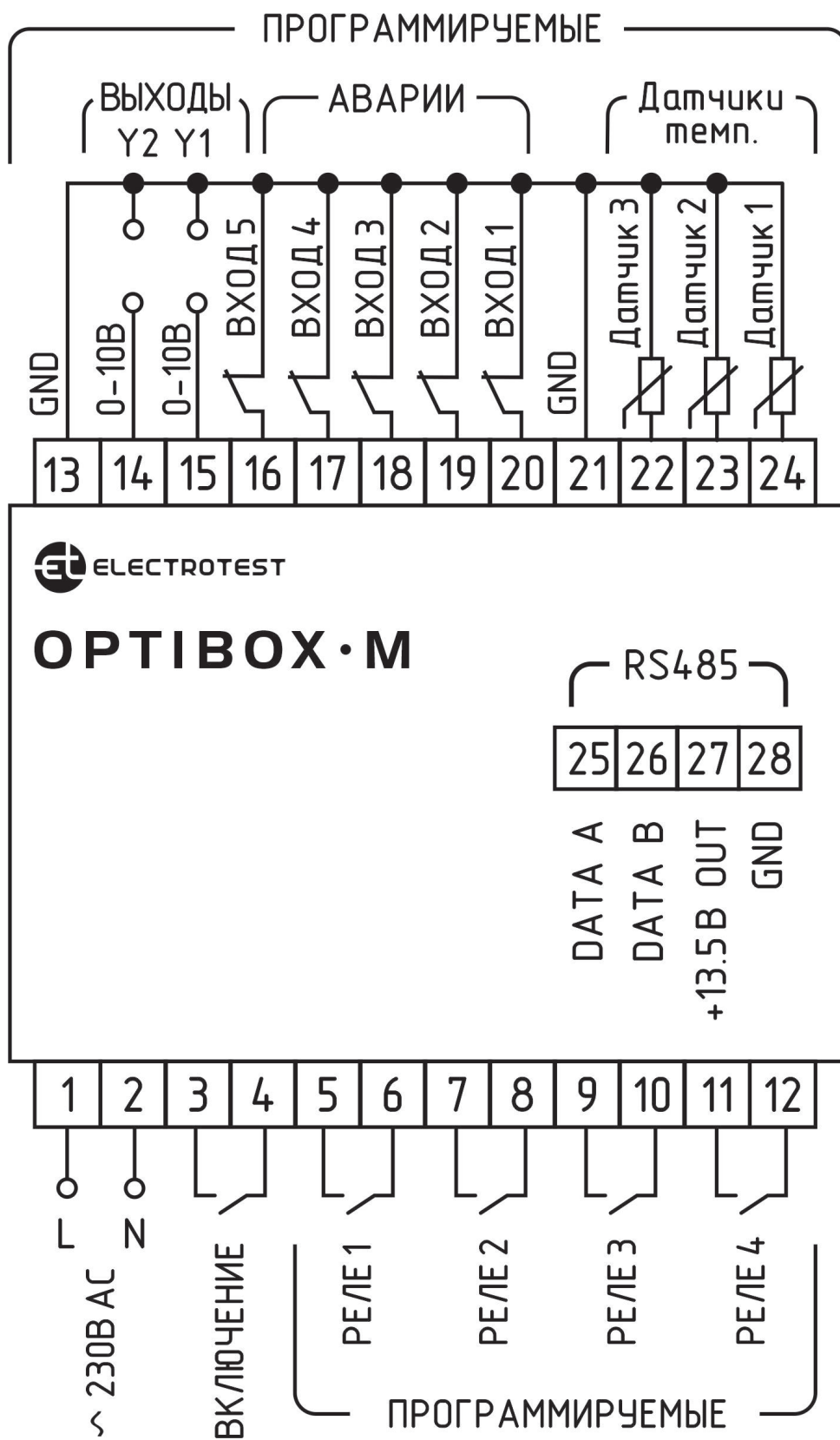
Рис. 2.1 Назначение клемм контроллера.
