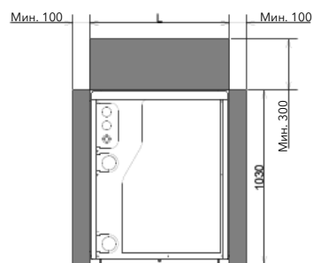
Вид спереди
