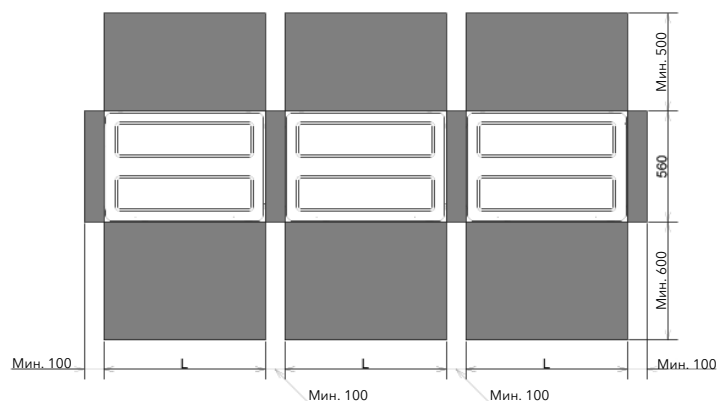
Вид сверху
