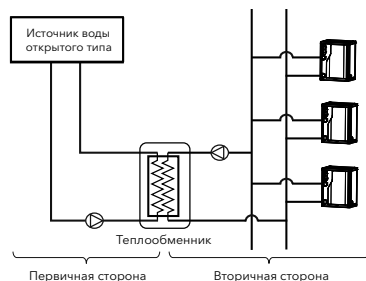
Водяной контур открытого типа с теплообменником
