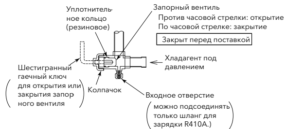
Теплонасосная система
