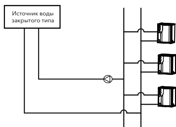
Водяной контур закрытого типа
