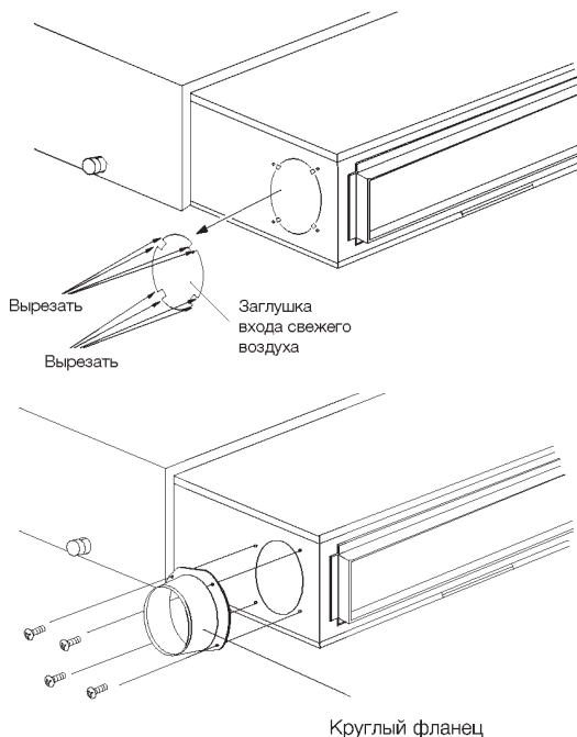
Круглый фланец
