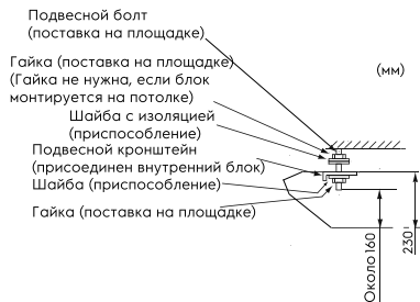
Для потолочной установки
