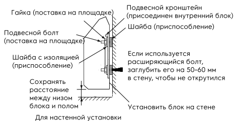
Для настенной установки
