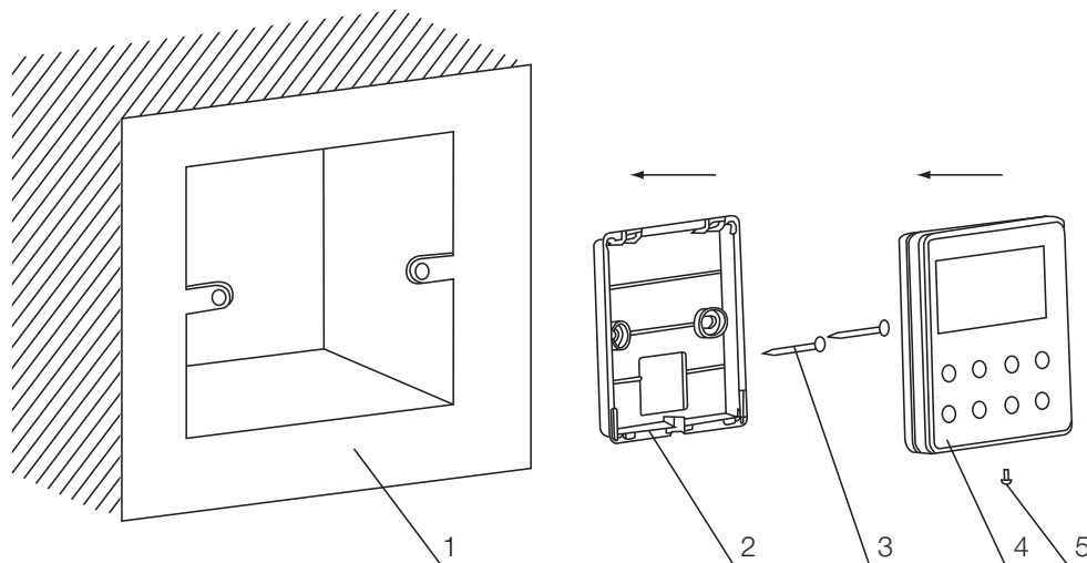
Схема установки проводного пульта
