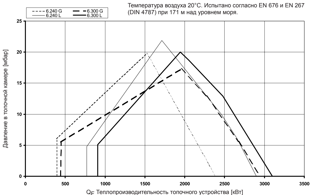
Рабочая зона EK 6.240 / 300 GL-EUF
