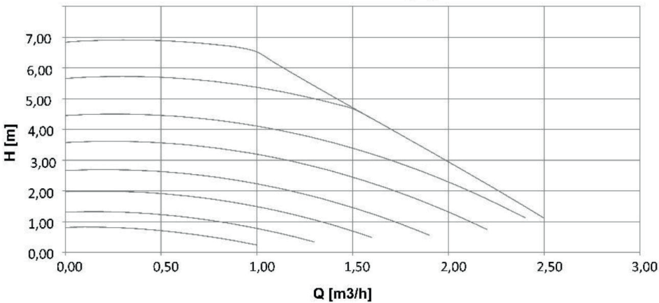
Кривая расхода - высоты напора
