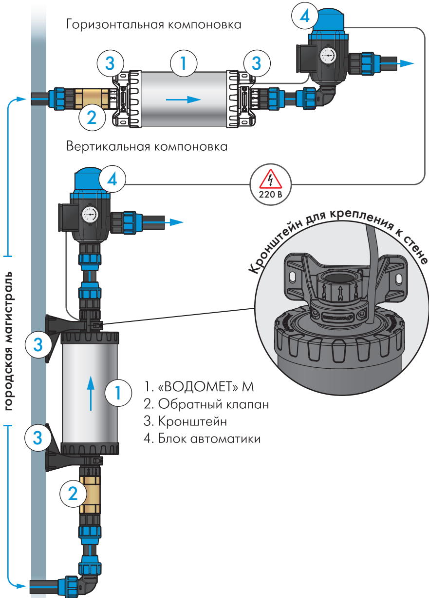
Рисунок 5. Пример установки магистрального насоса.
