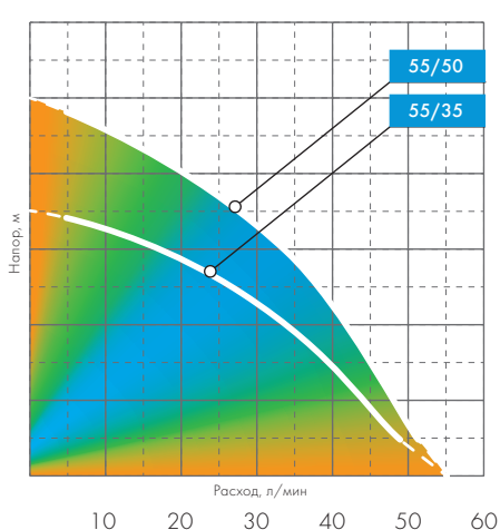
График расходно-напорных характеристик*:
