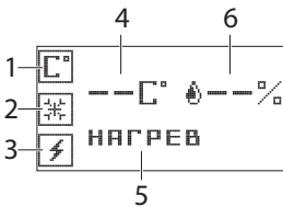
Рис. 7. Главный экран, нормальный режим
