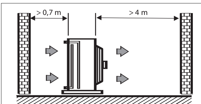
FLUSSO D'ARIA ORIZZONTALE HORIZONTAL AIR FLOW
