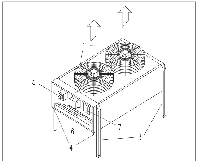
DISPOSIZIONE CON FLUSSO D'ARIA VERTICALE VERTICAL AIR DISCHARGE ARRANGEMENT
