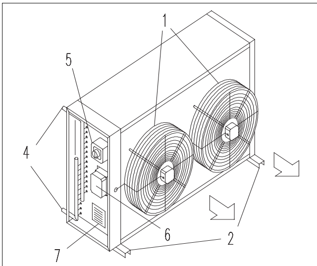
DISPOSIZIONE CON FLUSSO D'ARIA ORIZZONTALE HORIZONTAL AIR DISCHARGE ARRANGEMENT
