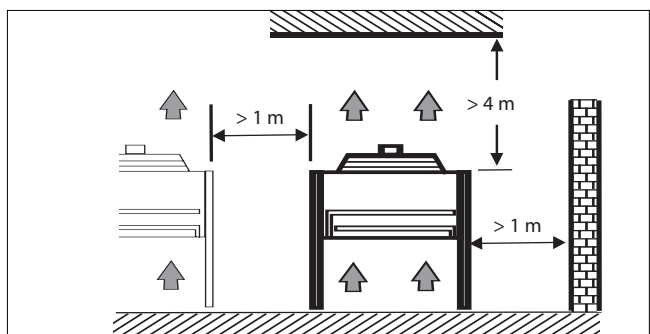
FLUSSO D'ARIA VERTICALE VERTICAL AIR FLOW
