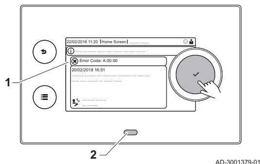
Рис. 39 Отображение кода ошибки на МКЗ
