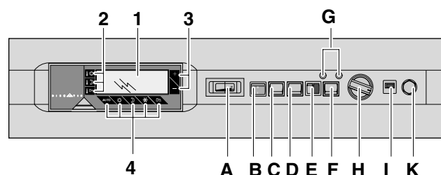
Панель управления DIEMATIC-m Delta 8358N002
