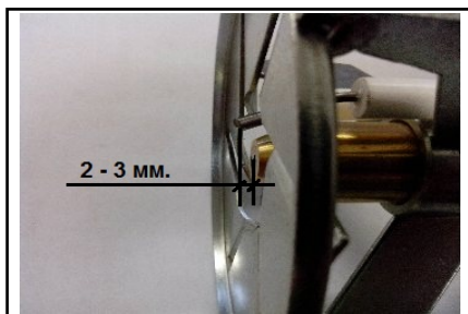
Форсуночный блок
