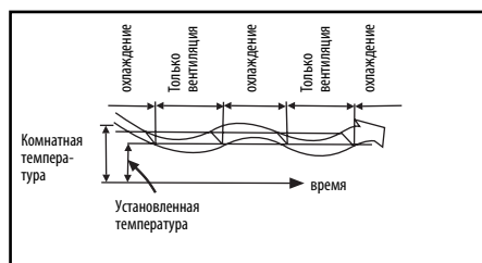
РЕЖИМ ОСУШЕНИЯ
